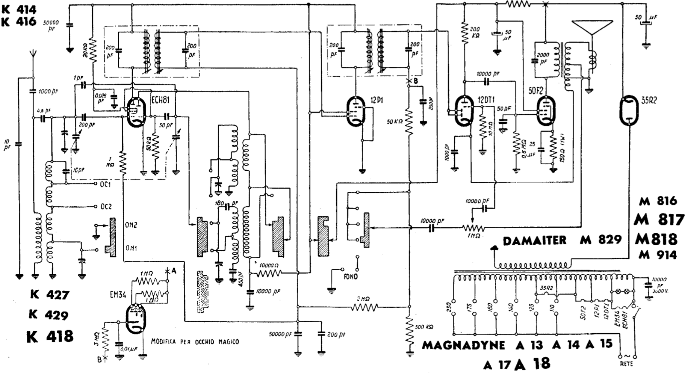
MAGNADYNE RADIO - Modd. MAGNADYNE A 13, A 15, A 18; KENNEDY K 418, K 427, K 429; DAMAITER M 818 ed M 829. Gamma onde medie suddivisa e due gamme onde cortc. Media frequenza 471 kc/s. I modelli Magnadyne A 18, Kennedy K 18 e Damaiter M 18 differiscono dagli altri modelli menzionati per avere l'occhio magico. I modd. Damaiter M 816, M 817, M 914; Kennedy K 414, K 416; Magnadyne A 14, A 16 e A 17 hanno le seguenti valvole: UCH42, 12BA6, 12AT6 e 50B5.
